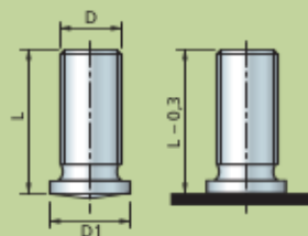
Goujons filetés "AT"
