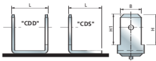
Cosses à souder "CDS" ou "CDD"
