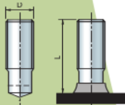
Goujons filetés à base réduite "BR"
