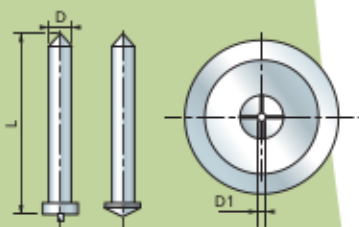
Clous d'isolation et clips "CD"
