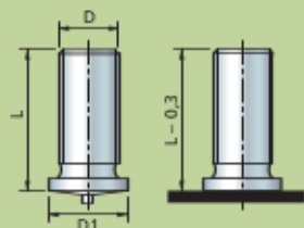
Goujons filetés "CD"
