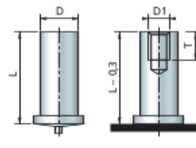
Douilles percées taraudées "CD"
