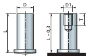
Douilles percées taraudées "AT"
